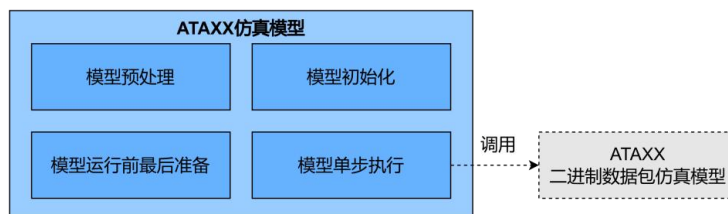
图 23 模型组成结构
