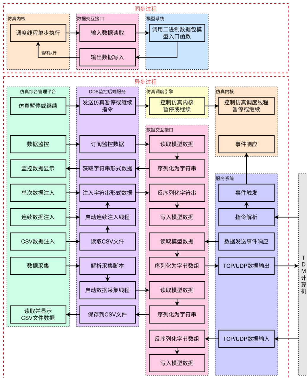
图 59 “玄鸟”架构仿真运行阶段处理流程
