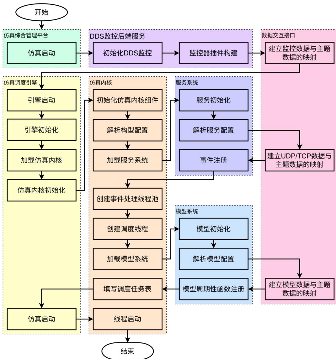
图 58 “玄鸟”架构仿真启动阶段处理流程
